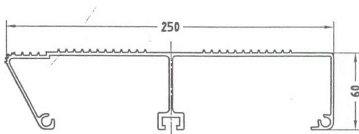
C - TRAPTREDEPROFIEL
